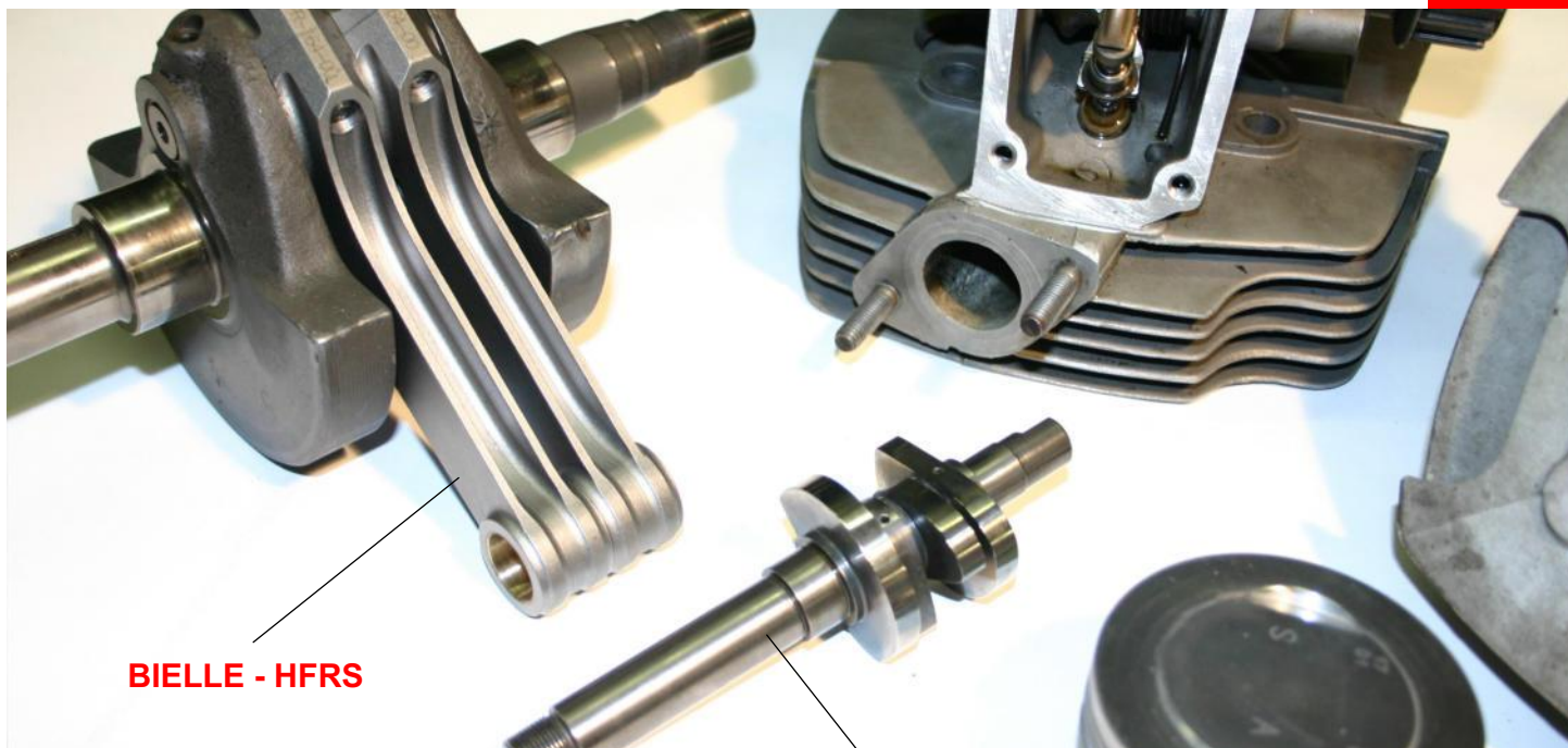
ALBERI A CAMME - DRAGON
